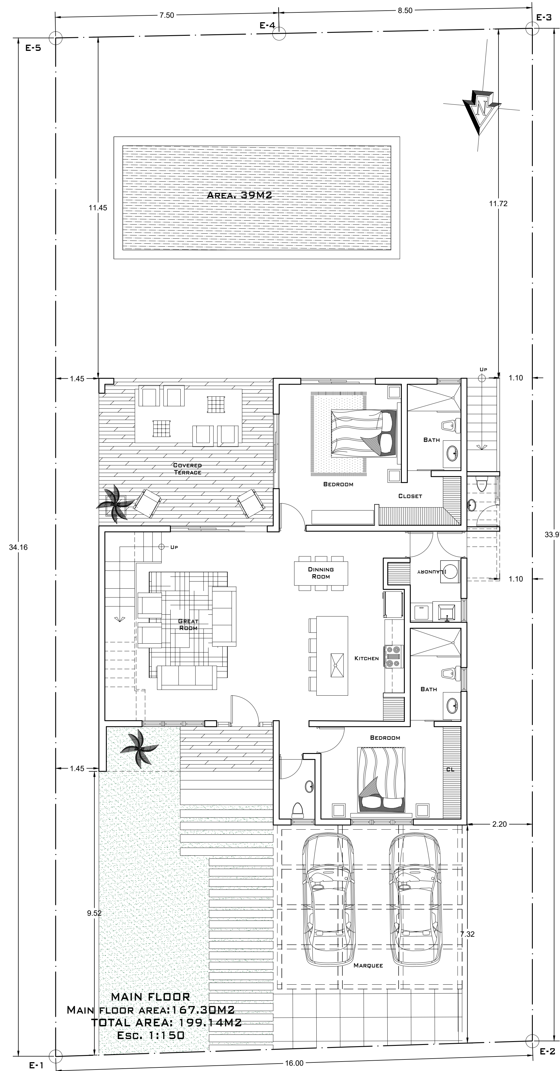
PLANTA ARQ. AMUEBLADA 1er Nivel Esc. 1:50
